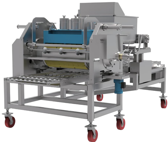
CMK-CX600 滚筒式全自动成型机
