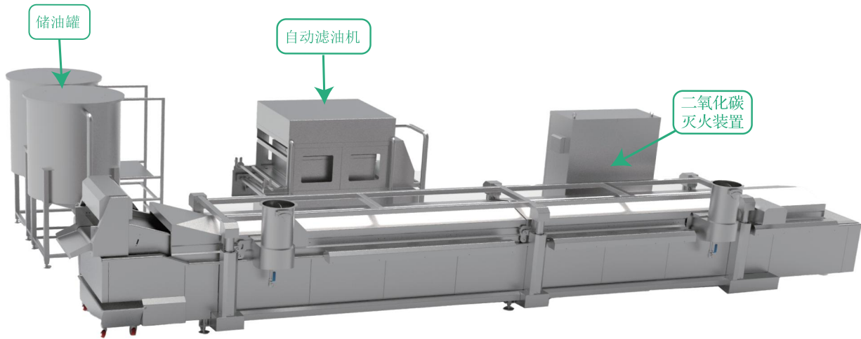
600mm宽油炸机参数表
